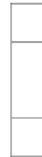
_art. 27/P _struttura colonna 3 vani _cm L 59 - P 36 - H 238,5
