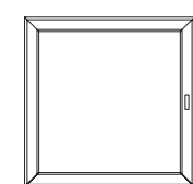
_art. 43/P _anta liscia per laccatura _cm L 59 - SP 2,7 - H 59
