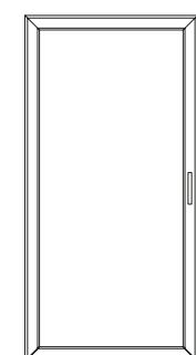
_art. 48/P _anta liscia per laccatura _cm L 59 - SP 2,7 - H 118
