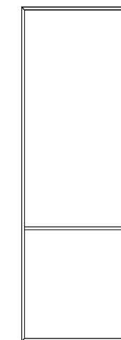
_art. 30/P _struttura colonna 2 vani _cm L 59 - P 36 - H 179,5
