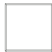
_art. 7/P _struttura base 1 vano _cm L 59 - P 36 - H 61,5
