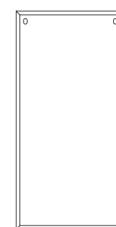
articolo SCM14 struttura pensile verticale 1 vano. cm. l. 59 - p. 36 - h. 118
