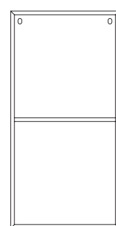
articolo SCM13 struttura pensile verticale 2 vani. cm. l. 59 - p. 36 - h. 118
