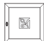
articolo EPS76 DX anta con intaglio per laccatura. cm. l. 59 - sp. 2,8 - h. 59
