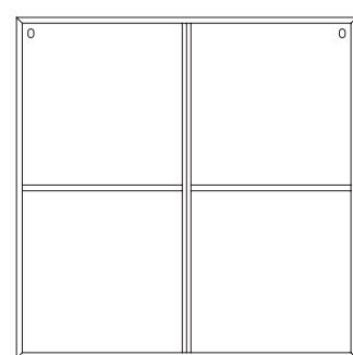
articolo SCM12 struttura pensile a cubo 4 vani. cm. l. 118 - p. 38 - h. 118
