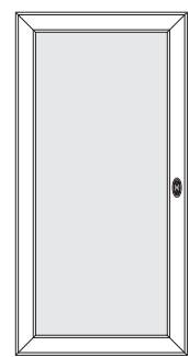
articolo SCM5 anta lunga per vetro. cm. l. 59 - sp. 2,8 - h. 118
