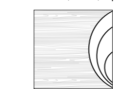
ART. CP/88 anta quadrata DX con incisioni laterali. cm. l. 58,6 h. 58,6 sp. 2,5
