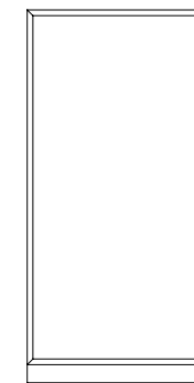
ART. CP/33 colonna 1 vano. cm. l. 59 p. 36 h. 124
