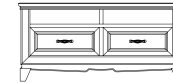
ART. SCM4 BASE porta TV 2 cassetti 2 vani a giorno. cm. l. 120,5 p. 55 h. 62
