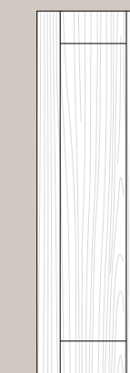
ART. CM38 anta a telaio legno verticale. cm. l. 36,6 h. 117,6 sp. 2,5
