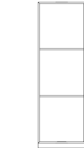
ART. CP/31 colonna 3 vani. cm. l. 59 p. 36 h. 183
