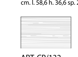
ART. CP/107 anta telaio verticale DX liscia. cm. l. 58,6 h. 117,6 sp. 2,5
