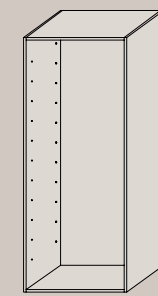
ART. CB1 FRASSINO ART. CB1 TANGANICA struttura cabina armadio doppia passo ripiani in h.16,7 cm. cm. 110 x 59 h.247
