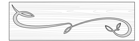
ART. EL/36SX anta con decoro orizzontale apertura vasistas cm. l.117,6 h.36,6 sp.2,5
