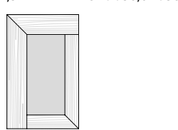
ART. CP/96 anta telaio verticale SX per vetri. cm. l. 36,6 h. 58,6 sp. 2,5
