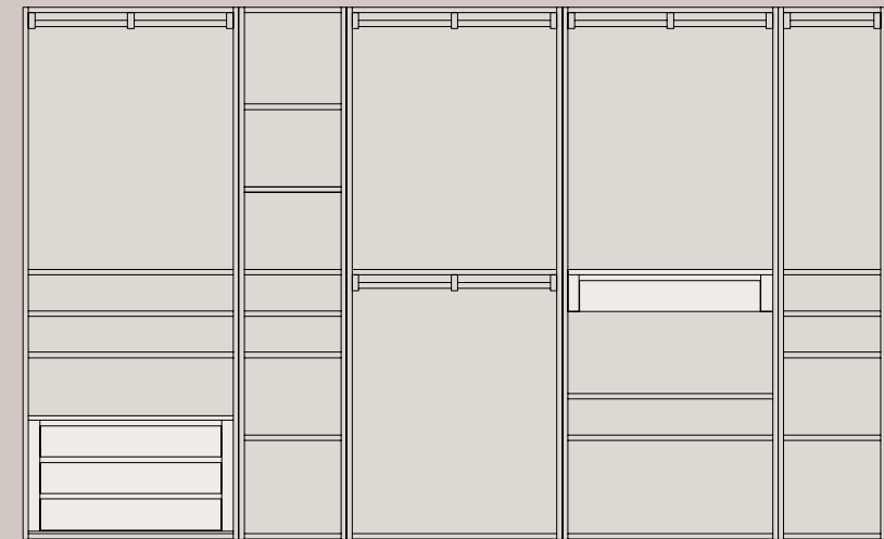
ART. 6128 proposta cabina armadio vista aperta. cm. l. 400 p. 59 h.247
