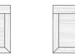
ART. CP/82 anta telaio quadrata DX liscia. cm. l. 58,6 h. 58,6 sp. 2,5
