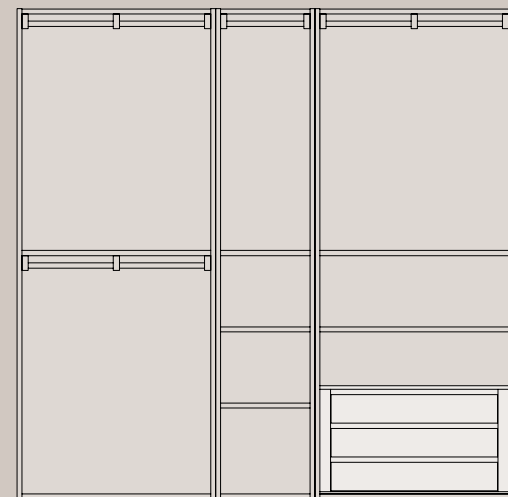
ART. 6133 proposta cabina armadio vista aperta. cm. l. 250 p. 59 h.247
