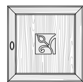
ART. EPS79 SX ANTA con intaglio per finitura noce. cm. l. 59 sp. 2,8 h. 59
