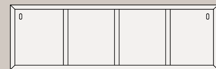
ART. EL/58 pensile libreria orizzontale cm. l.118 p.36 h.37
