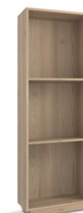
ART. E 88/SX - E 89/DX COLONNA in FRASSINO 3 vani. cm. l. 59 p. 36 h. 182,7
