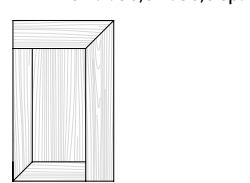
ART. CP/95 anta telaio verticale DX liscia. cm. l. 36,6 h. 58,6 sp. 2,5
