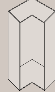
ART. CB52 FRASSINO ART. CB52 TANGANICA struttura angolo 90° 2 ante passo ripiani in h.16,7 cm. cm. 111,8 x 111,8/59 h.247
