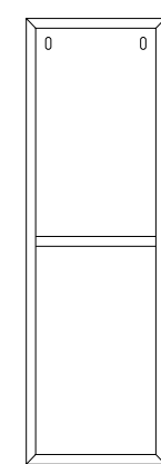
ART. CM18 pensile verticale 2 vani. cm. l. 37 p. 36 h. 118
