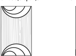
ART. CP/98 anta verticale con incisioni. cm. l. 36,6 h. 58,6 sp. 2,5
