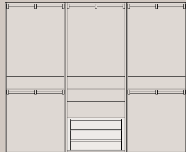
ART. 6132 proposta cabina armadio vista aperta. cm. l. 300 p. 59 h.247
