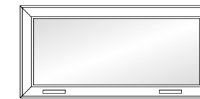
ART. C37/P PENSILE anta vetro apertura a vasistans. cm. l. 110 p. 37 h. 57
