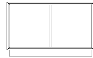
ART. C34/P BASE con 2 ante. cm. l. 110 p. 37 h. 66
