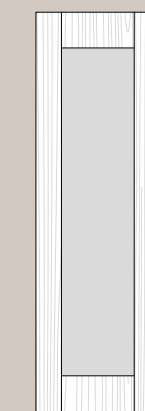
ART. CM39 anta a telaio vetro verticale. cm. l. 36,6 h. 117,6 sp. 2,5
