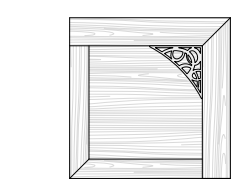
ART. CP/80 anta telaio quadrata DX con traforo. cm. l. 58,6 h. 58,6 sp. 2,5
