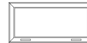
ART. C37/A/P PENSILE anta legno a vasistans. cm. l. 110 p. 37 h. 57
