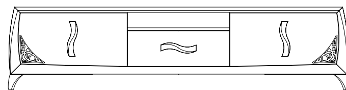
ART. CP/14 base 3 cestoni con traforo e vano. cm. l. 248 p. 57 h. 60
