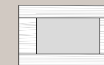
ART. CM36 anta a telaio vetro orizzontale vasistas. cm. l. 58,6 h. 36,6 sp. 2,5
